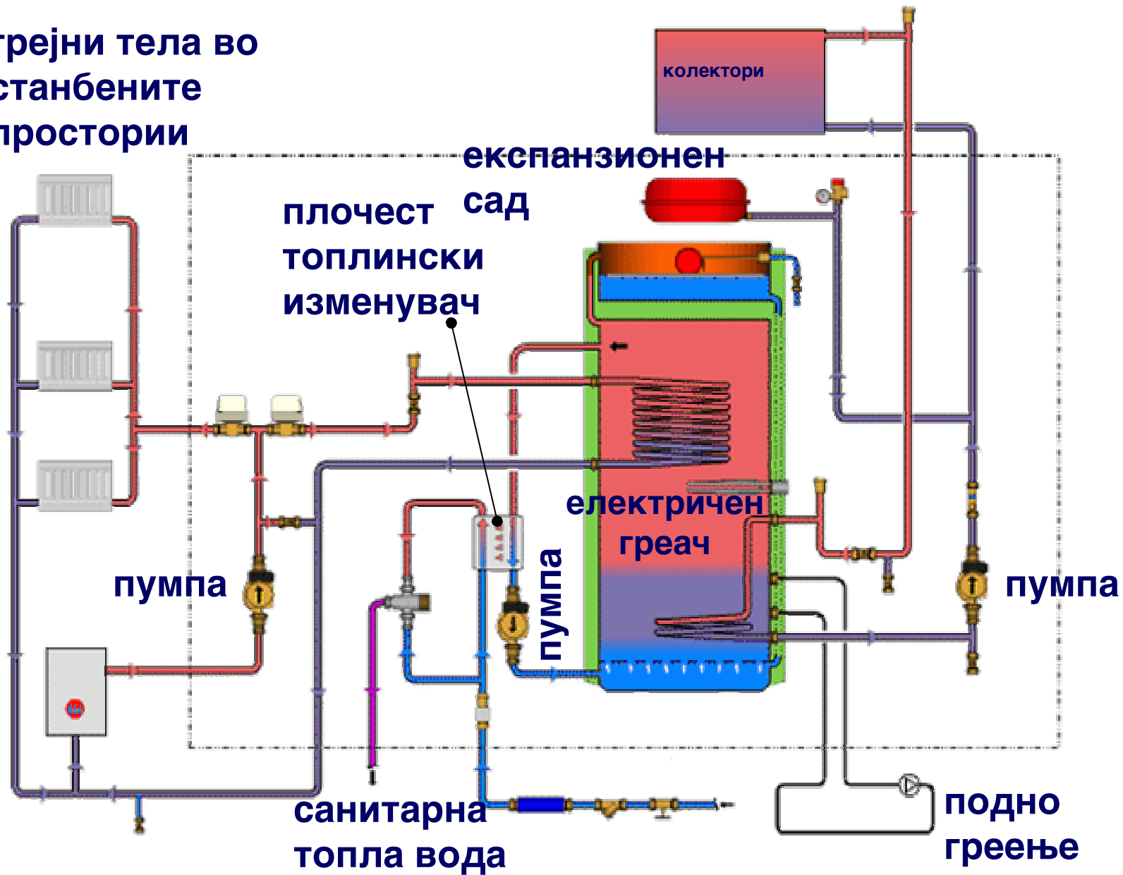
Комби систем со електричен греач
